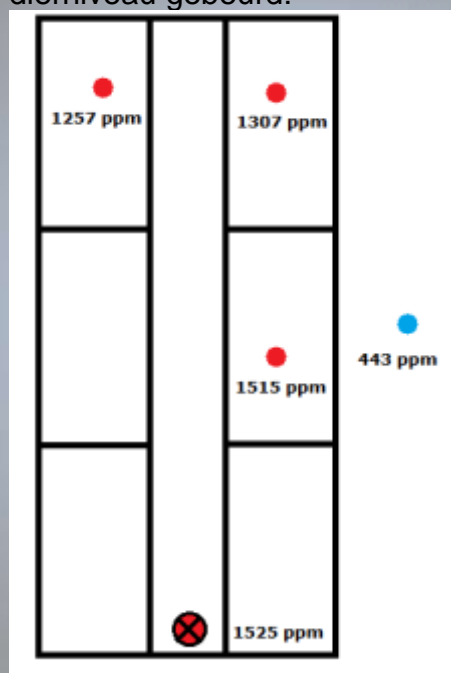
Figuur 9 Plattegrond CO 2 -metingen
