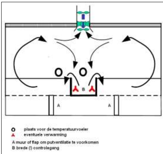
Figuur 1 Doorsnede deurventilatie (bron: Klimaatplatform varkenshouderij)
