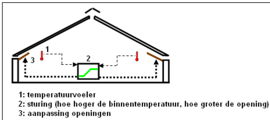
Figuur 10 Sturing bij natuurlijke ventilatie
