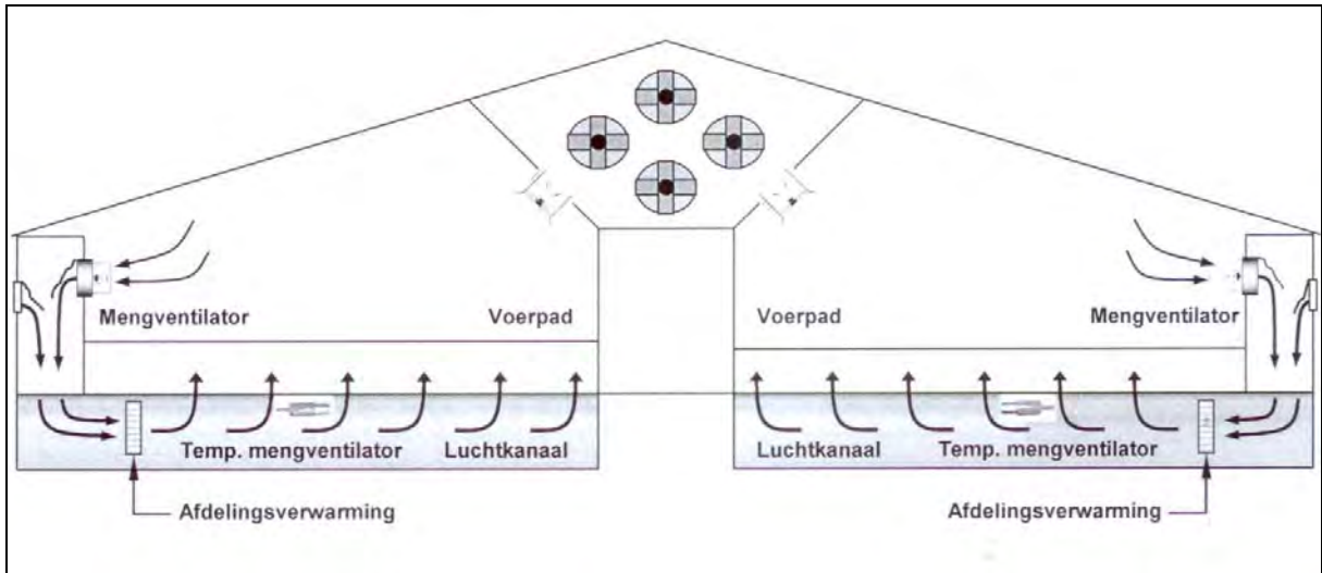
Figuur 43 Mengventilatie
