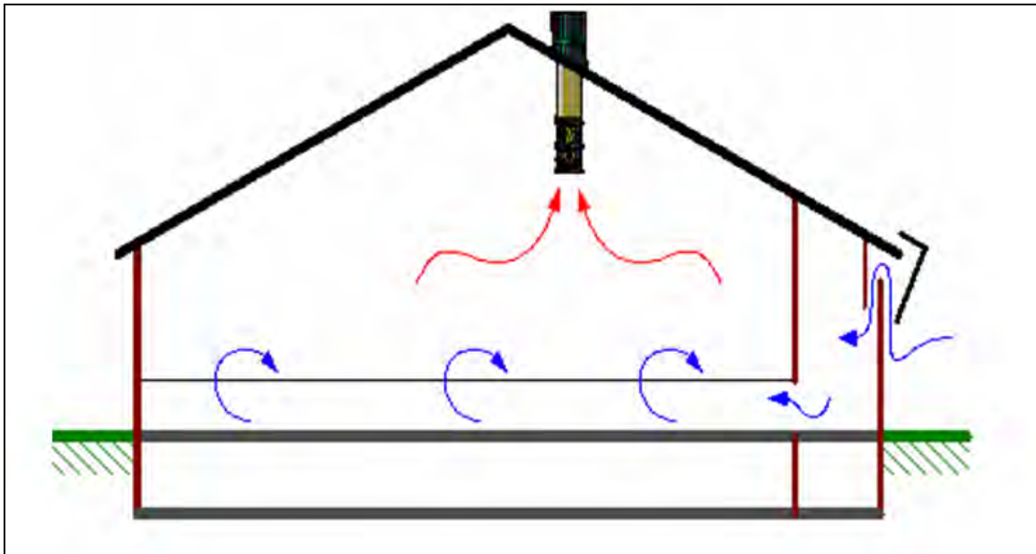
Figuur 19 Schema deurventilatie (Bron: Fancom)
