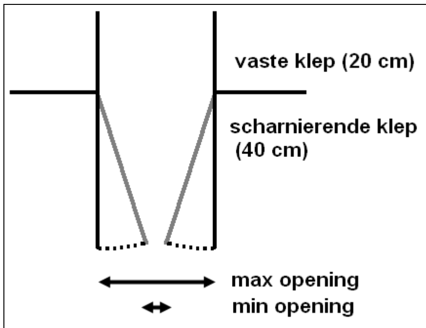
Figuur 31 De onderste klep dient regelbaar te zijn
