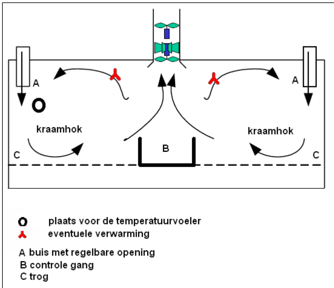
Figuur 37 Doorsnede buisventilatie in een kraamafdeling (bron: Klimaatplatform varkenshouderij)
