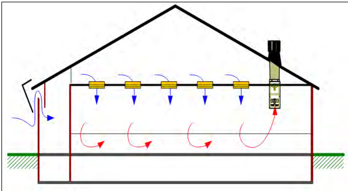
Figuur 27 Schema plafondventielventilatie (Bron: Fancom)
