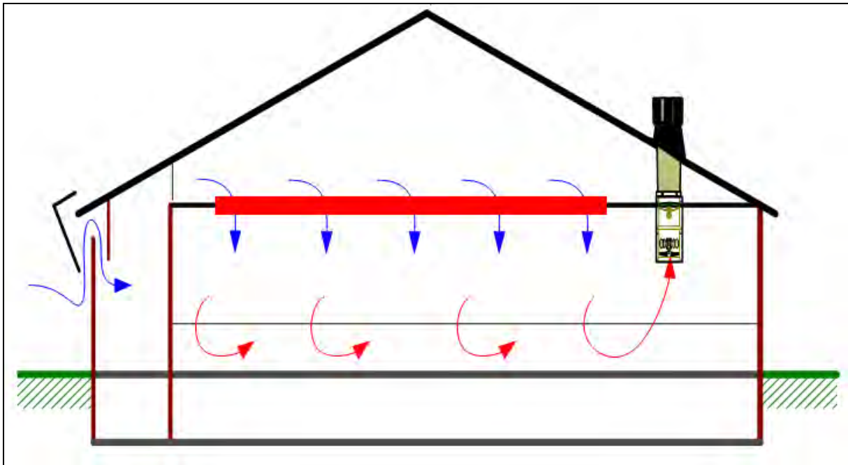
Figuur 29 Schema combiventilatie (Bron: Fancom)
