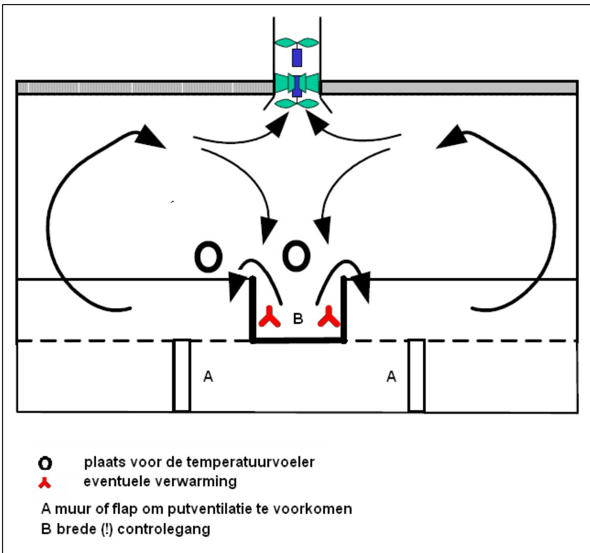
Figuur 20 Doorsnede deurventilatie (bron: Klimaatplatform varkenshouderij)
