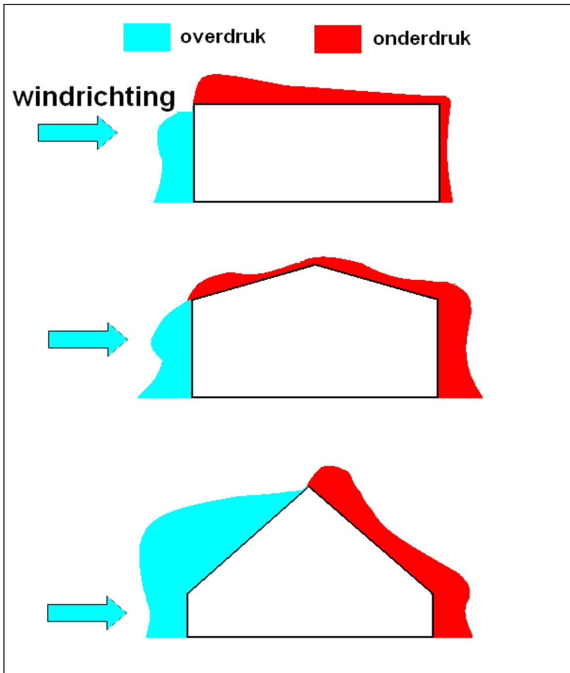
Figuur 9 Onderdruk en overdruk in functie van windrichting en staldoorsnede
