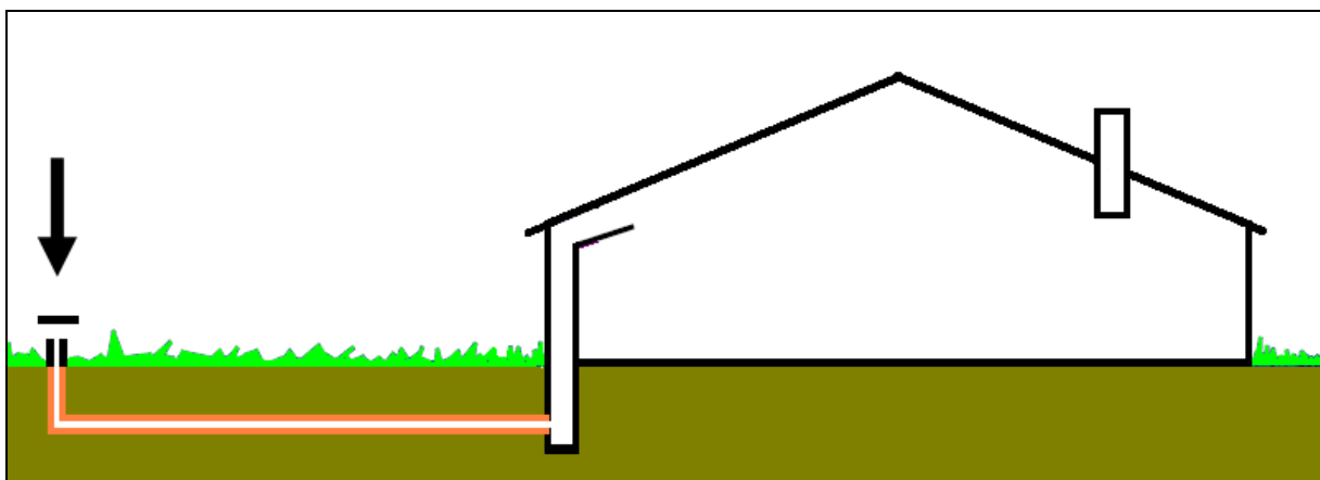
Figuur 42 Doorsnede grondbuisventilatie
