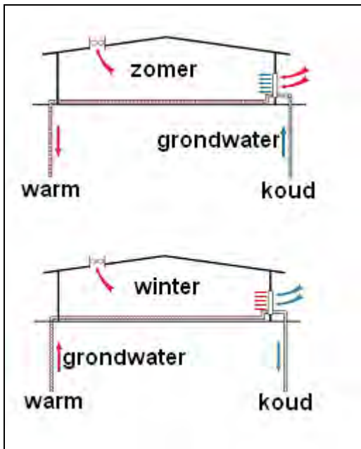
Figuur 41 Warmte-opslag in de bodem
