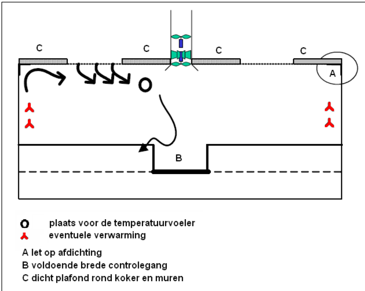
Figuur 24 Doorsnede plafondventilatie (Bron: Klimaatplatform varkenshouderij)
