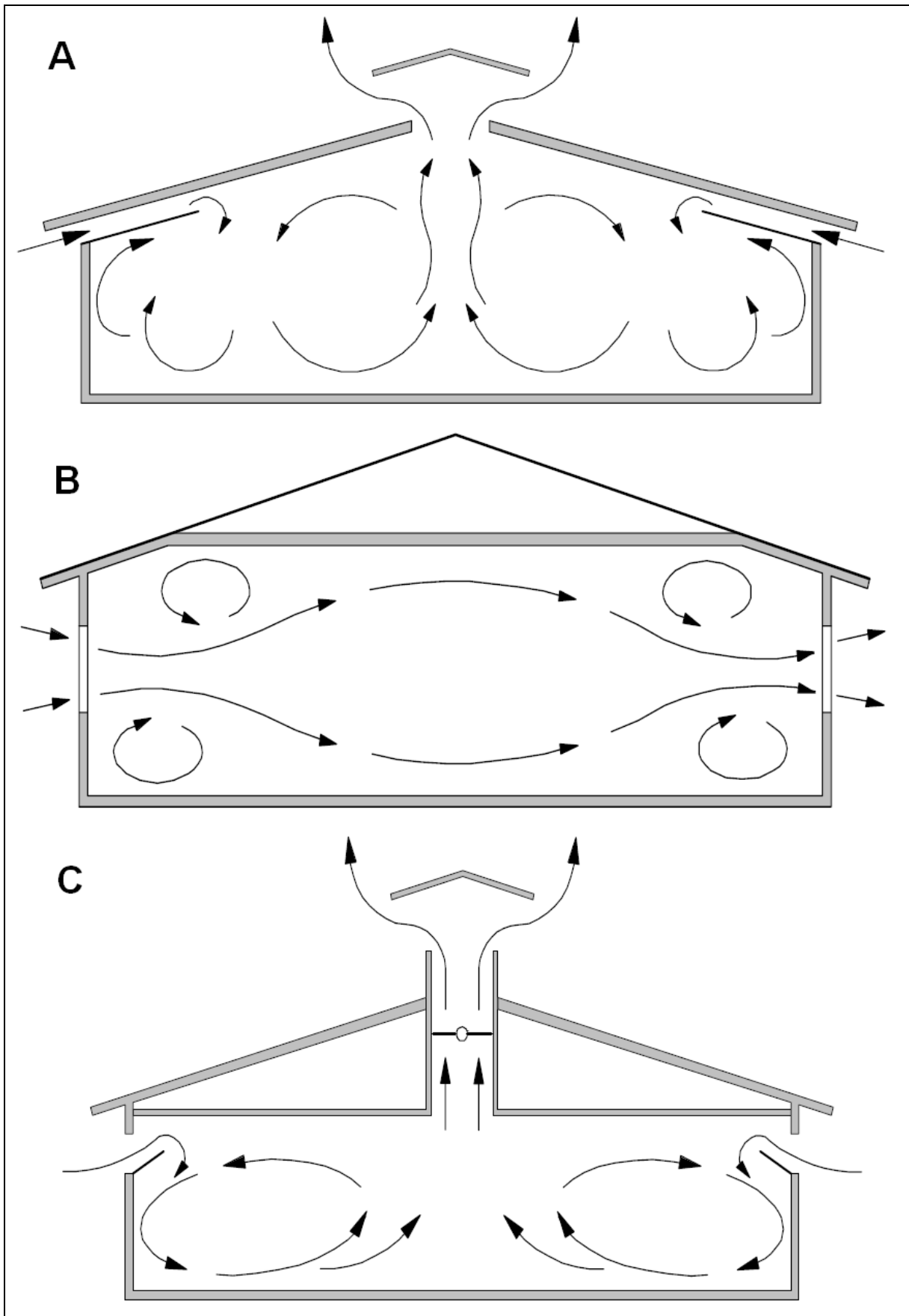
Figuur 8 De drie effecten aan de basis van een drukverschil A schoorsteeneffect, B windeffect en C ventilatoreffect (Bron: DLG)
