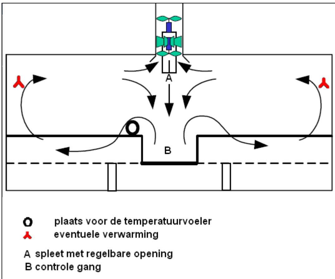
Figuur 30 Doorsnede combiventilatie (Bron: Klimaatplatform varkenshouderij)
