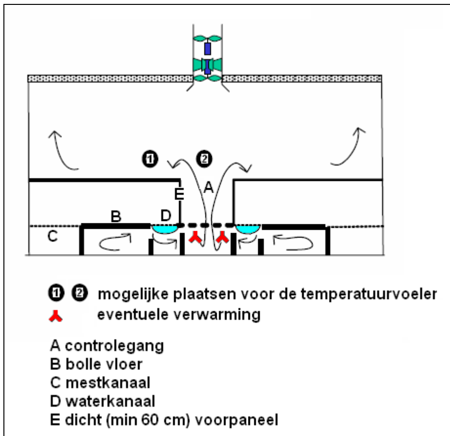
Figuur 34 Doorsnede kanaalventilatie via controlegang (bron: Klimaatplatform varkenshouderij)
