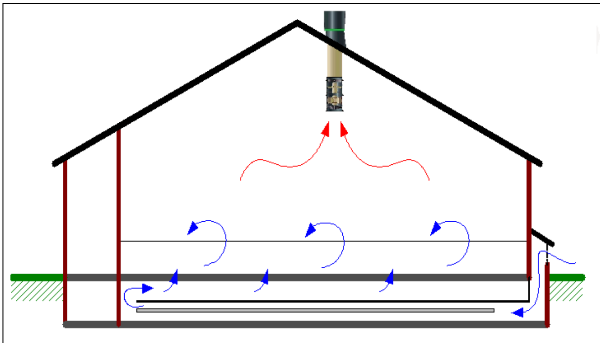
Figuur 33 Schema kanaalventilatie (Bron: Fancom)
