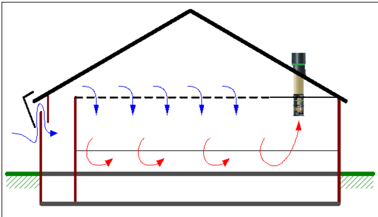
Figuur 25 Schema plafondventilatie (Bron:Fancom)
