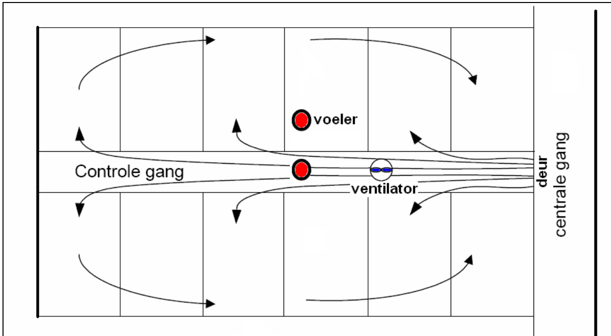
Figuur 21 Plattegrond in het geval van deurventilatie (bron: Klimaatplatform varkenshouderij)
