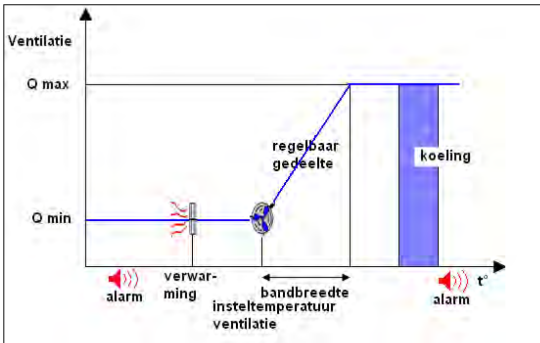
Figuur 5 Ventilatiegrafiek
