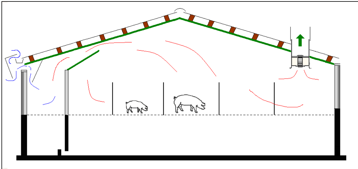
Figuur 14 Doorsnede klepventilatie (Bron: EMI)
