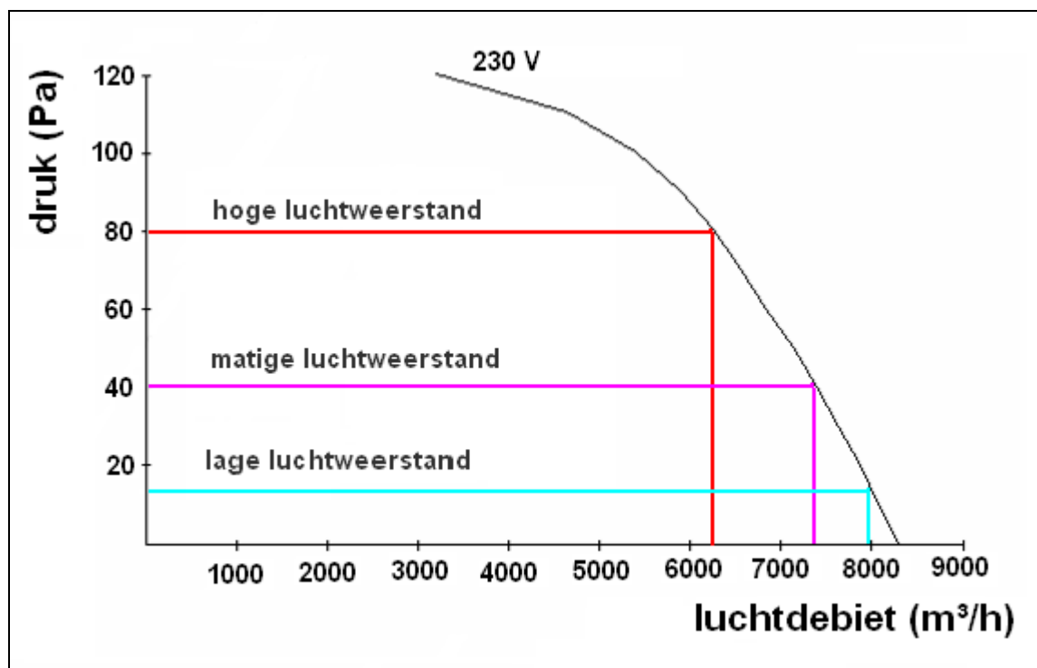
Figuur 6 Ventilatorspecifieke grafiek
