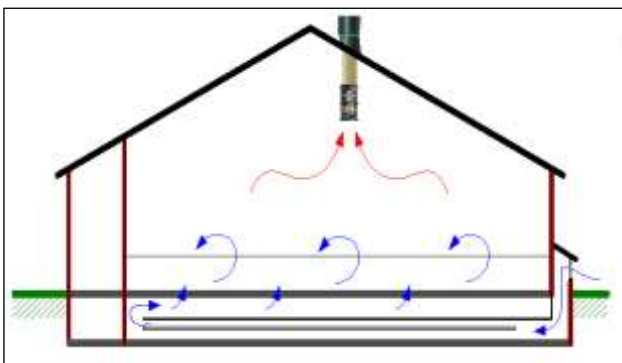
Figuur 1 Schema kanaalventilatie (bron: Fancom)
